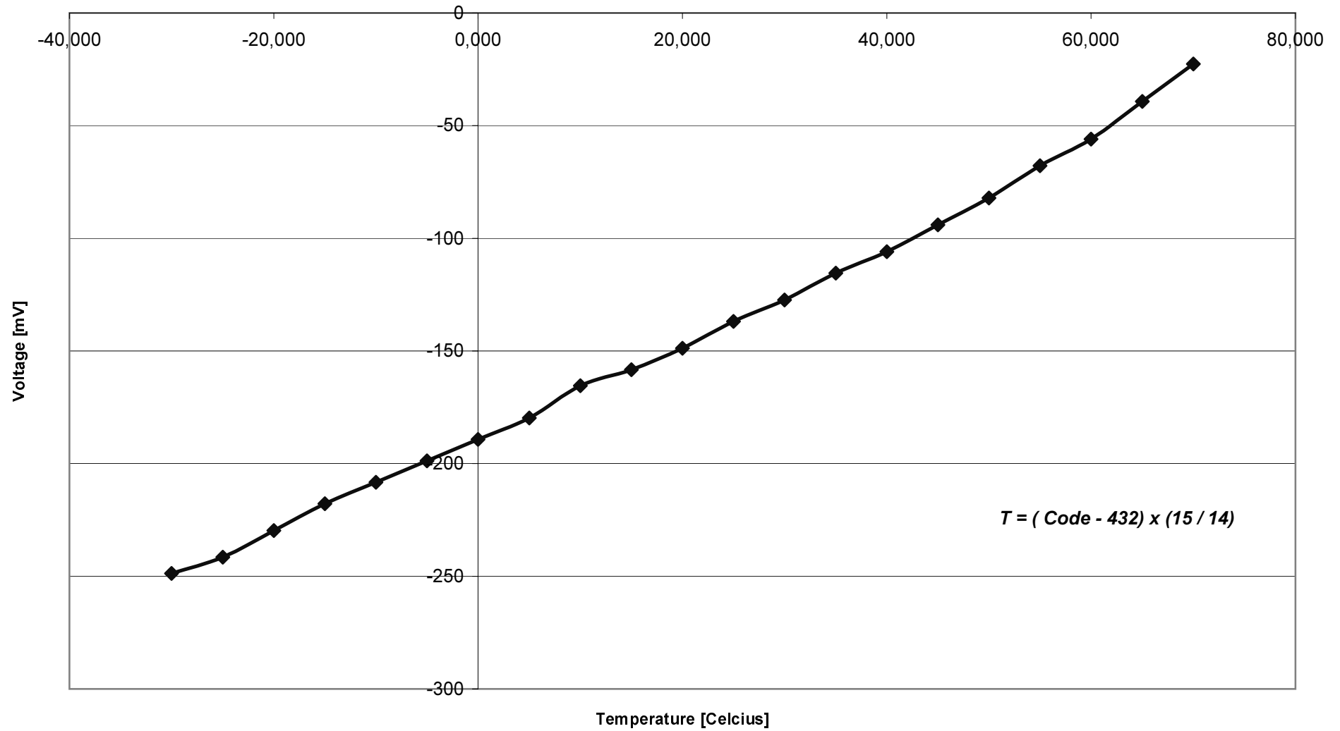
Temp-Sensor
